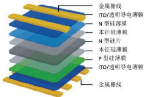
HDT太阳能电池芯片结构
